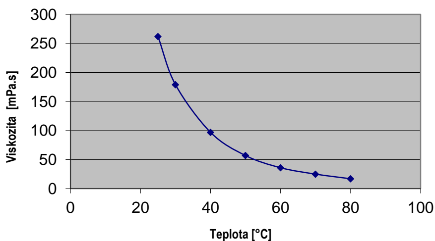
Závislosť viskozity NH 91 LV/u od teploty
